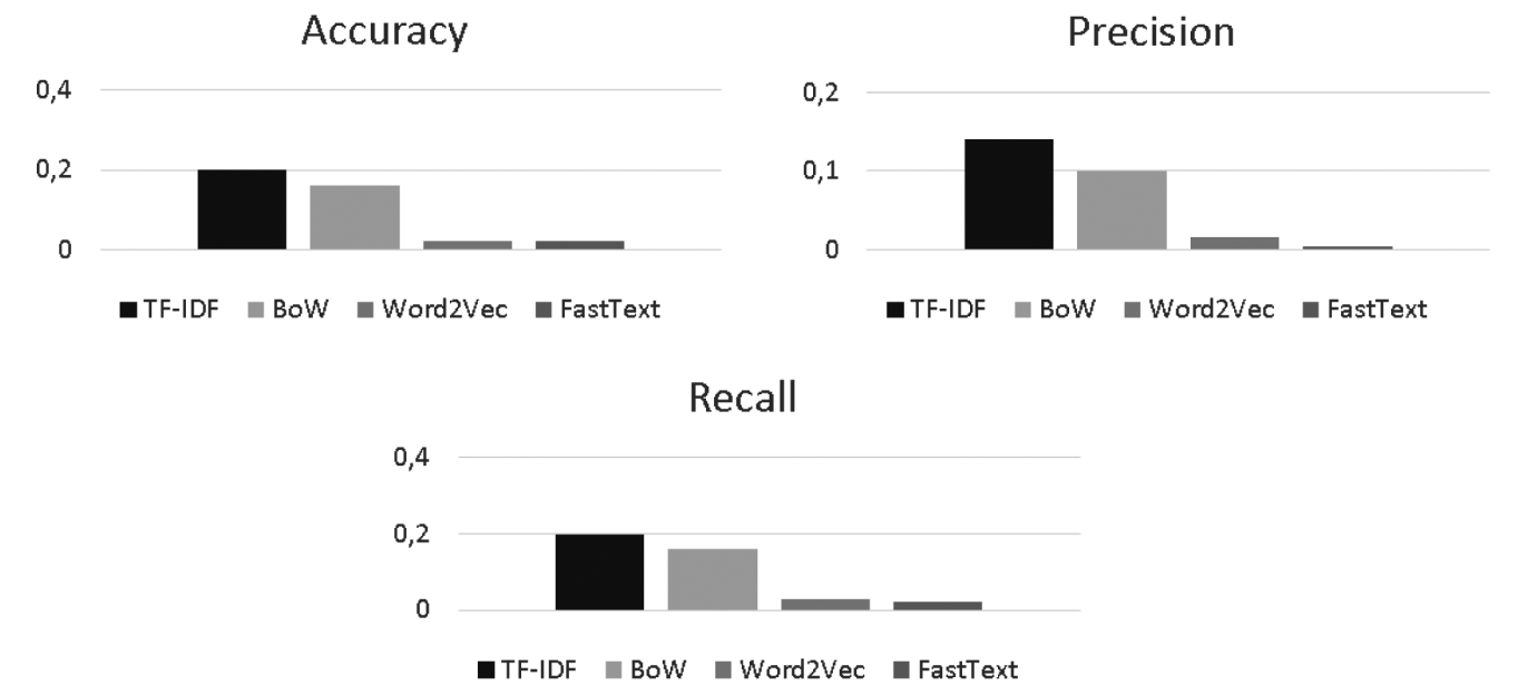
Рис. 1. Результаты метрик Accuracy, Precision и Recall
