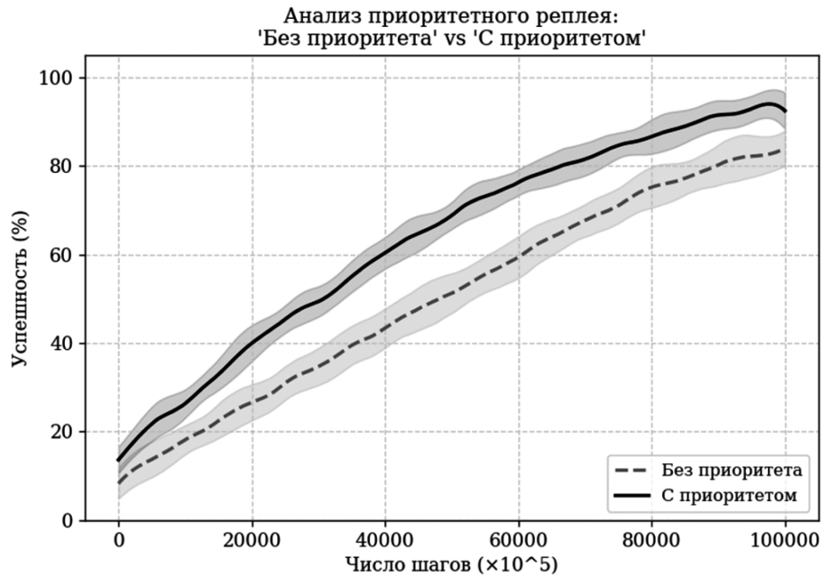
Рис. 7. Анализ приоритетного реплея: «Без приоритета» vs «С приоритетом» Сравнение нескольких алгоритмов по 4 метрикам
