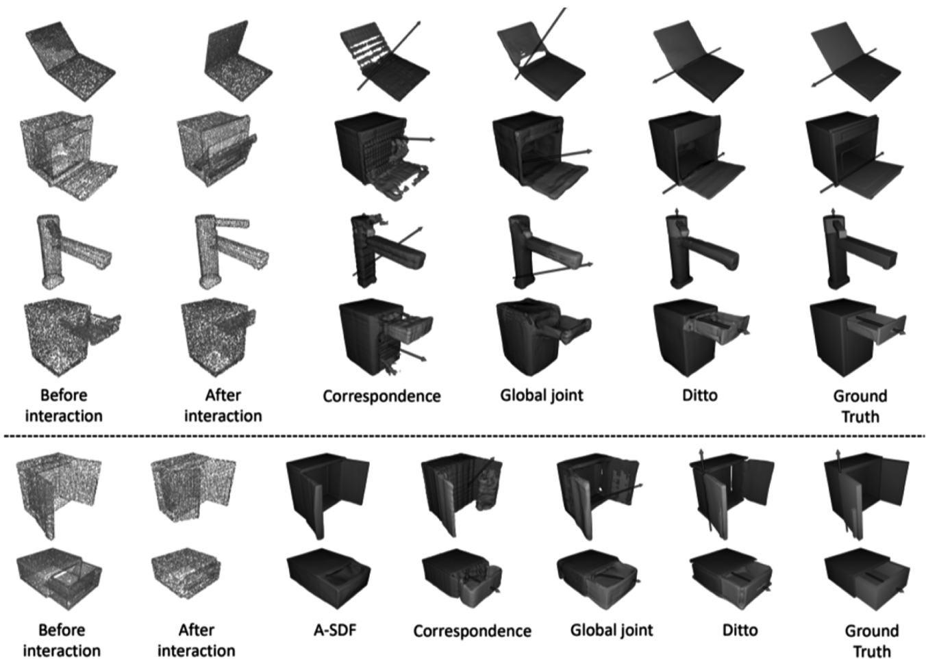
Рис. 4. Представлены результаты реконструкции ранее не наблюдаемых сочлененных объектов [12]
