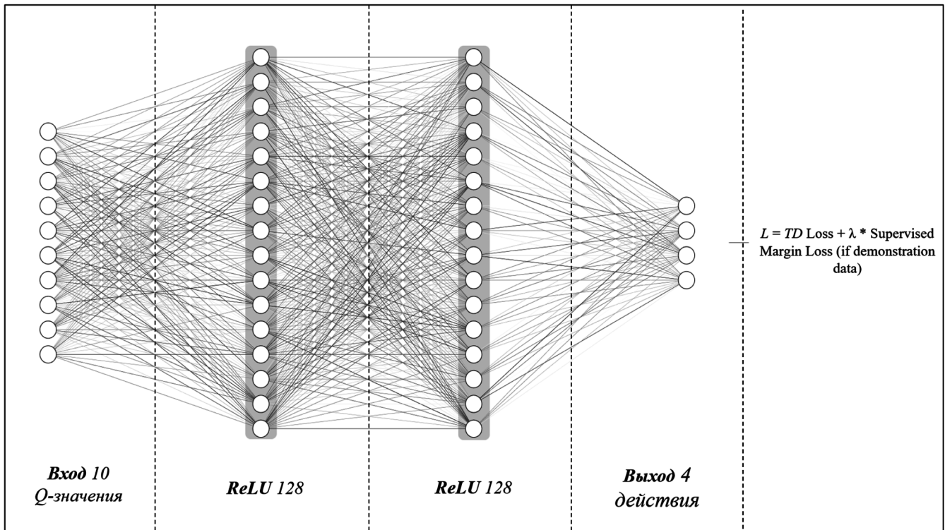
Рис. 3. Архитектура сети (двухслойная MLP с 128 нейронами в каждом скрытом слое)
