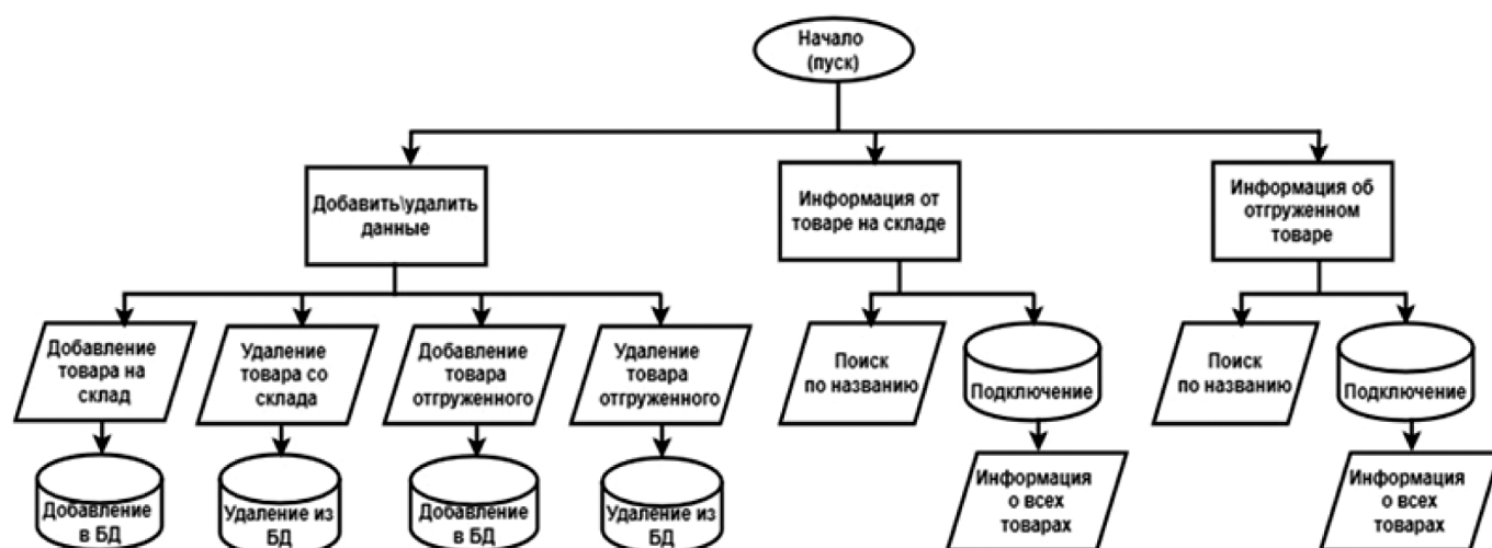
Рис. 2. Блок-схема консольного приложения
