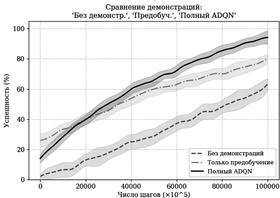
Рис. 6. Сравнение демонстраций: «Без демонстраций», «Только предобучение», «Полный ADQN»
