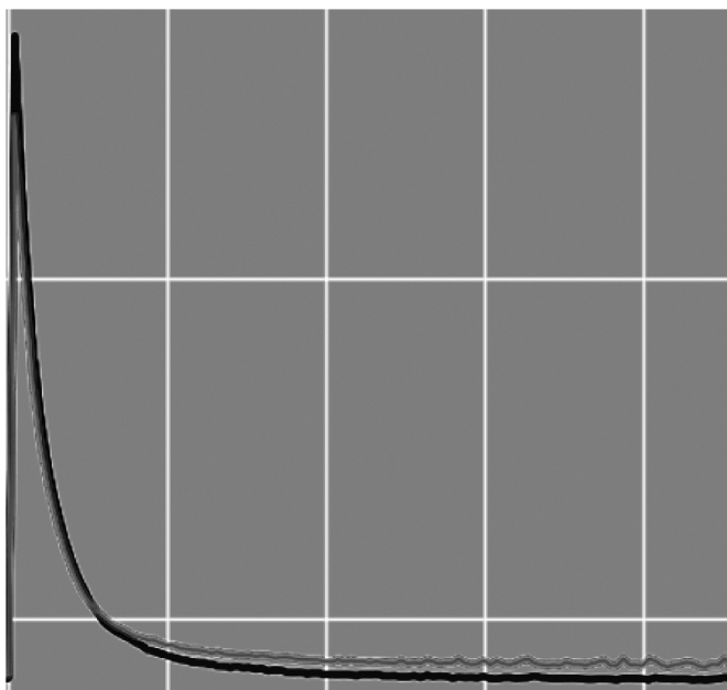
Рис. 6. Итоговые кривые обучения и валидации
