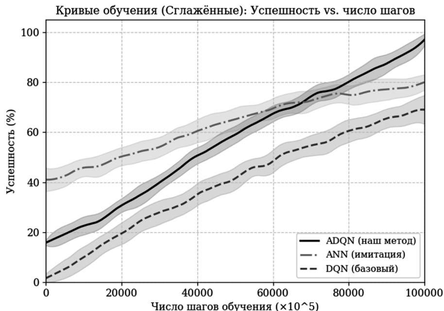
Рис. 5. Кривые обучения (ADQN, ANN, DQN): преимущество ADQN как на ранних этапах, так и по конечной успешности
