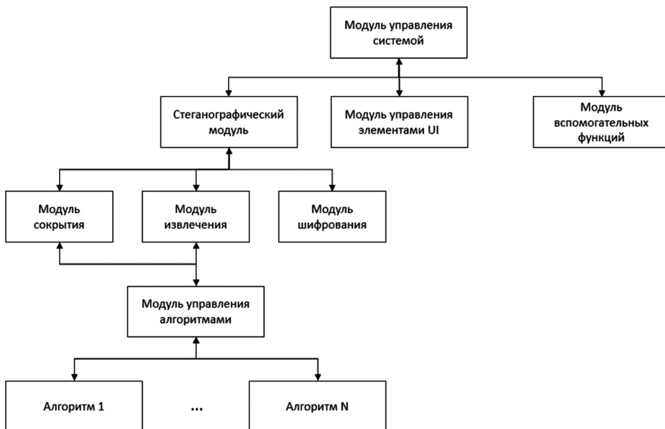
Рис. 1. Блок-схема архитектуры программного комплекса
