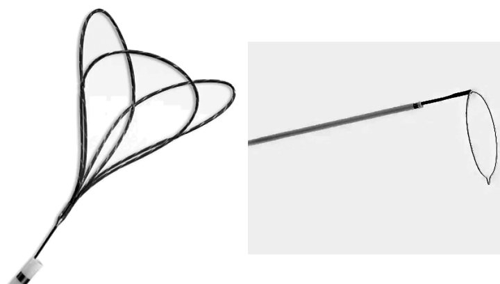
Рис. 1. (фото из интернета). Эндоваскулярная петля-ретривер one snare. Позолоченная петля из вольфрама и нитинола сохраняет круглую форму, обеспечивающую захват инородных тел. Нитиновый сердечник с памятью формы и высокой упругостью для поддержки при навигации по сосудам
