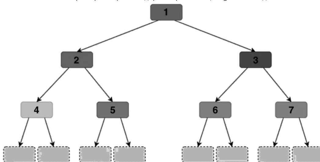
Рис. 2. Пример построения дерева при помощи XGBoost модели
