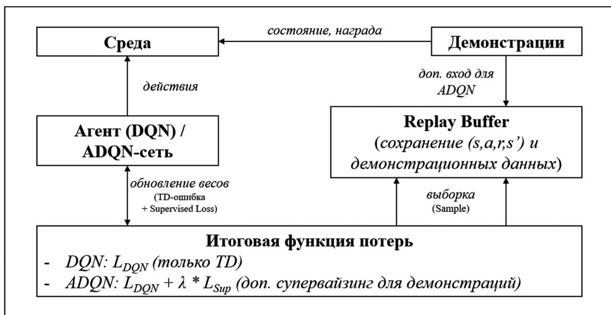
Рис. 1. Обобщённая блок-схема. Разница DQN (только TD-ошибка) и ADQN (TD + супервизия по действиям эксперта)
