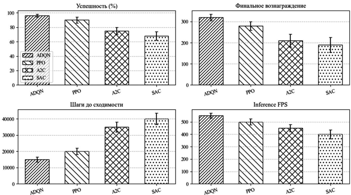
Рис. 8. Сравнение нескольких алгоритмов (PPO, A2C, SAC) по четырём метрикам. ADQN показывает преимущество как по успеху и вознаграждению, так и по скорости сходимости.
