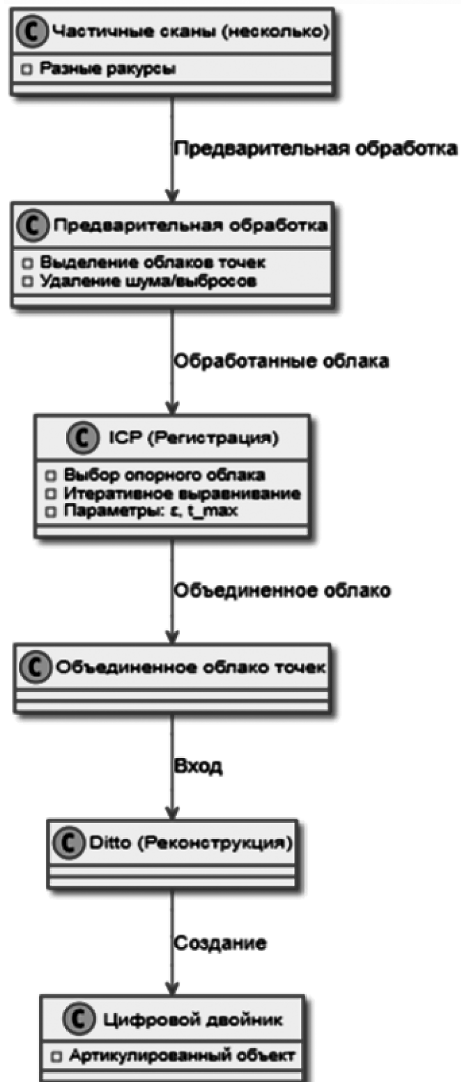
Рис. 5. Схема применения алгоритма ICP в процессе создания цифровых двойников
