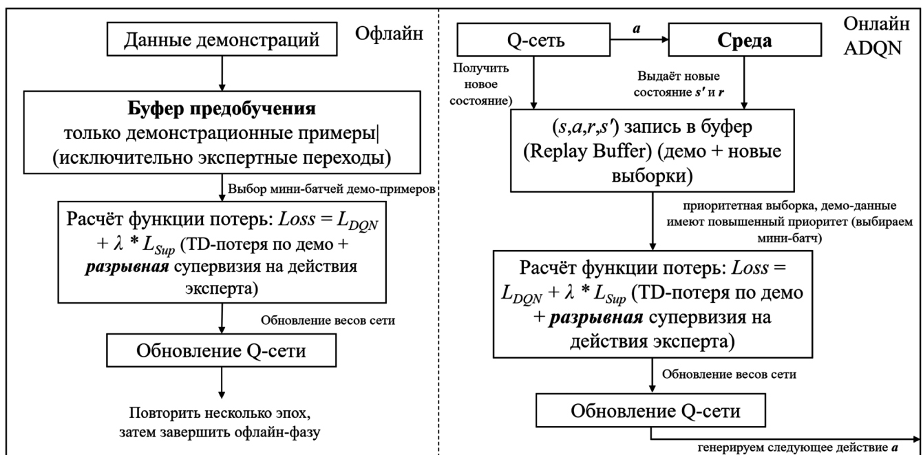
Рис. 2. Общая схема обучения ADQN
