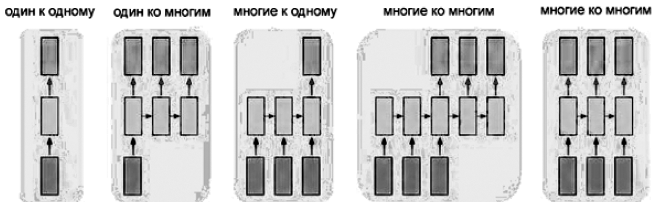
Рис. 3. Виды RNN
